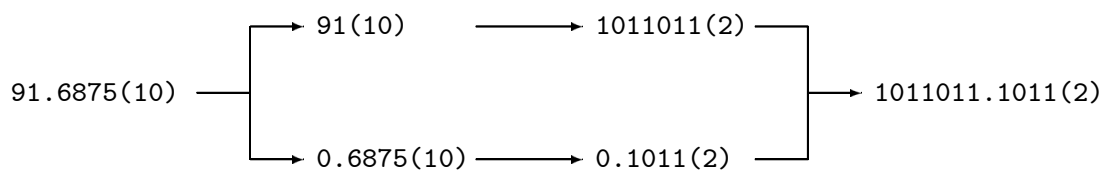
図 2.1: 整数部及び小数部を含む数の基数変換
