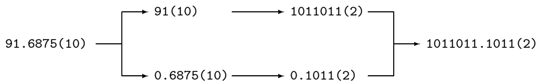
図 2.1: 整数部及び小数部を含む数の基数変換
