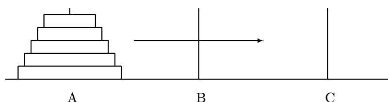
図 5.1: ハノイの塔
